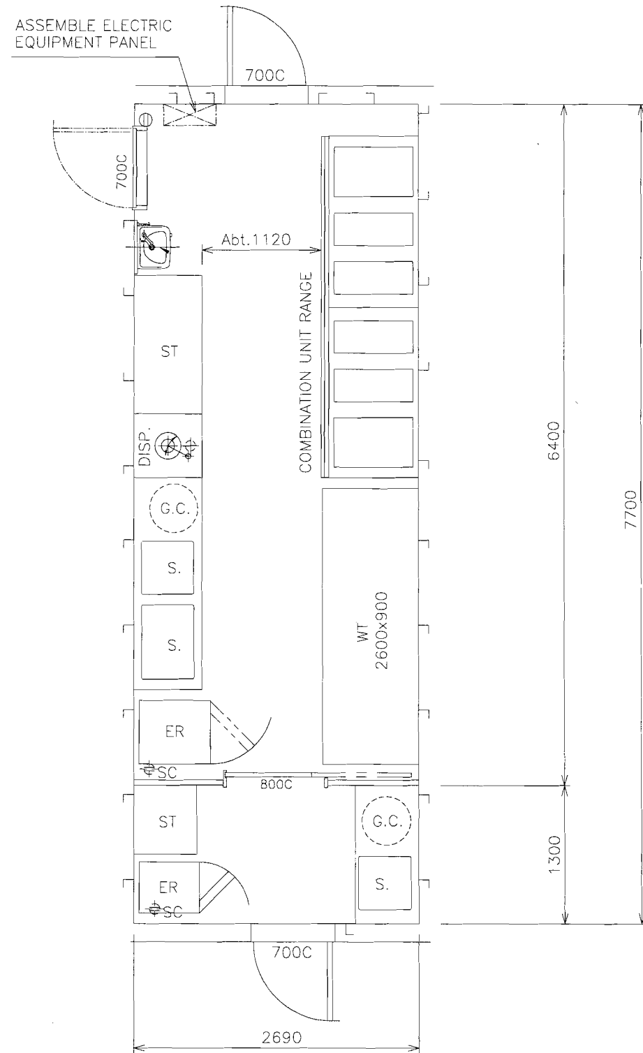
PLAN "A" 大型船用
